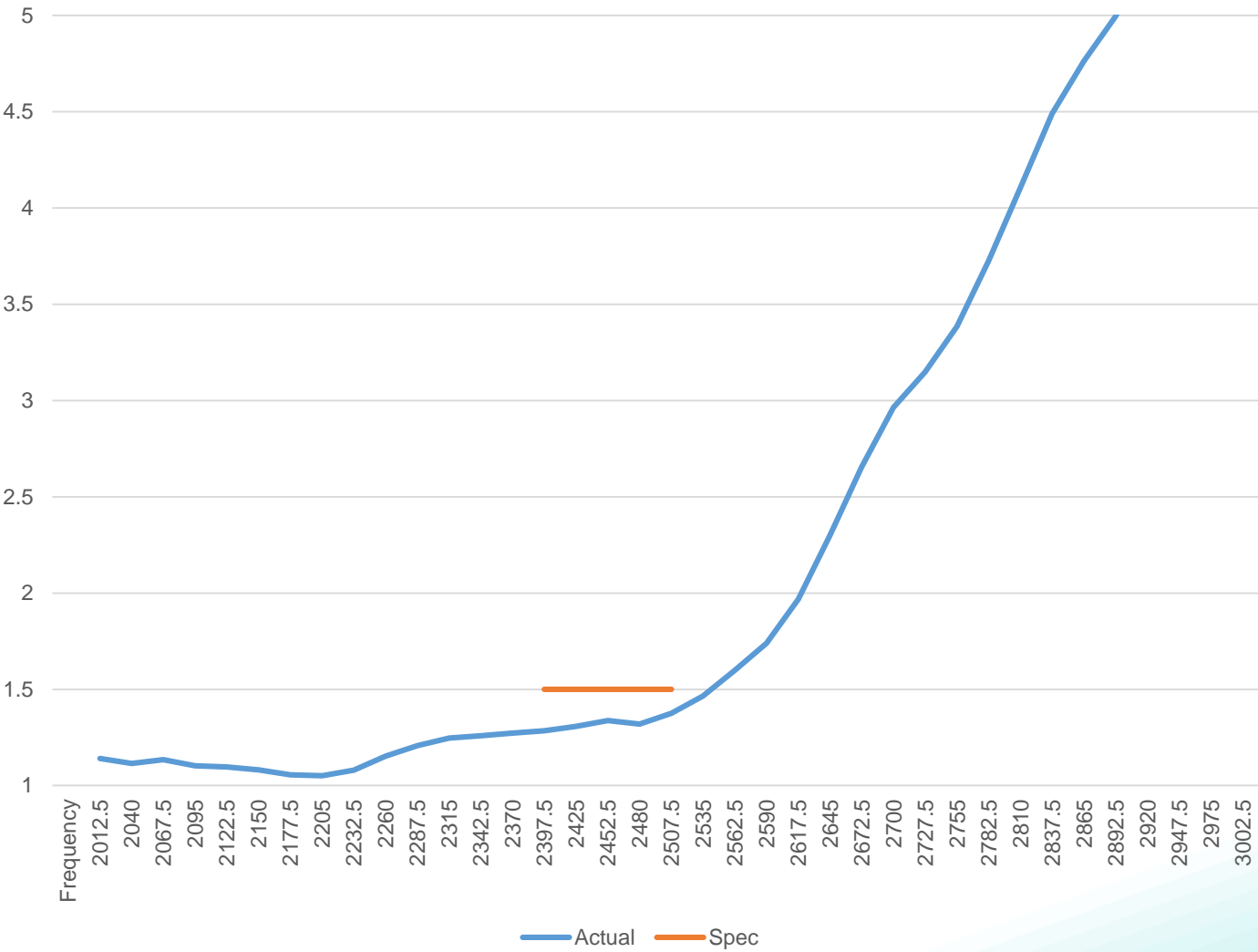
ICEFIN24NMOHF VSWR
