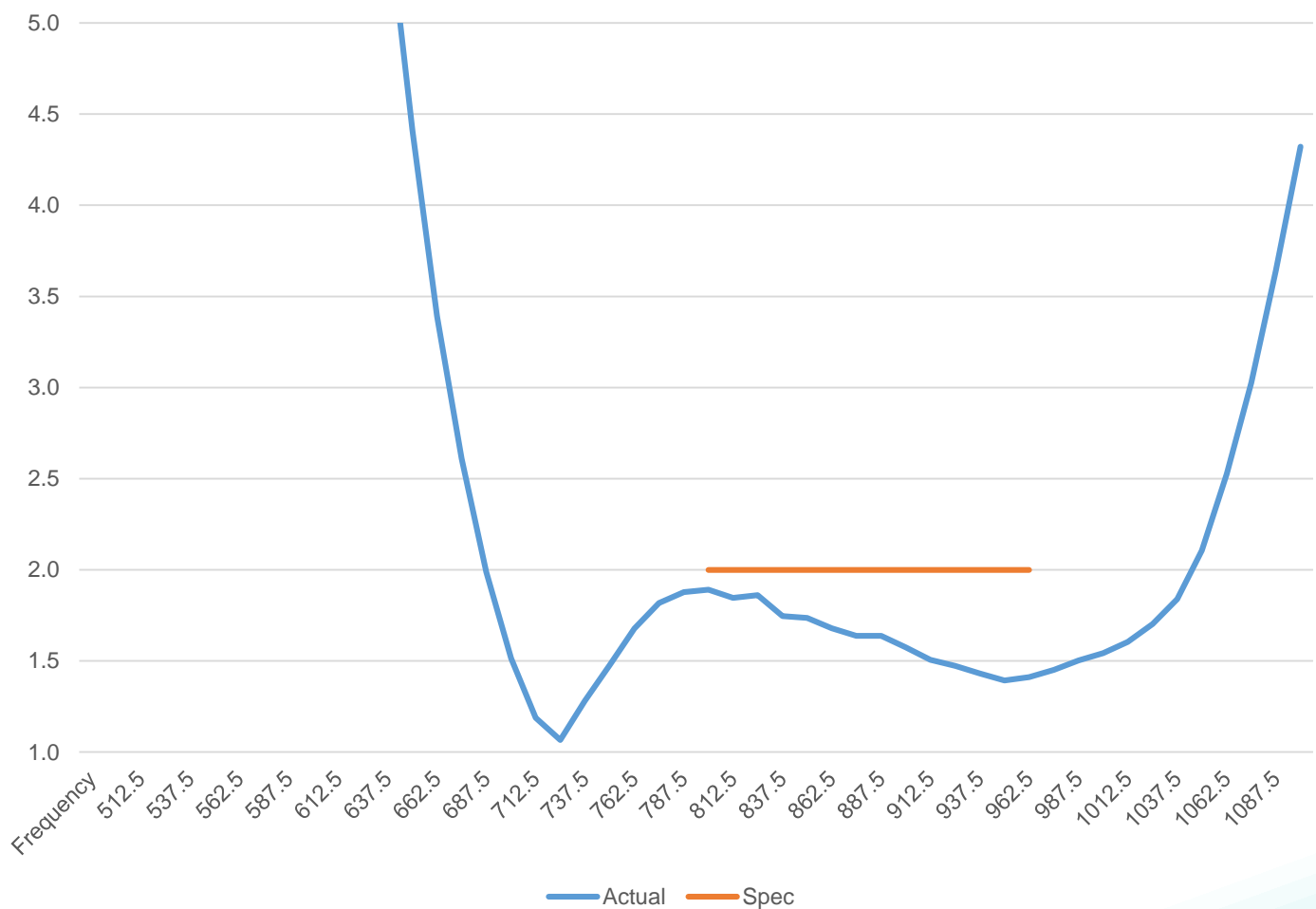
ICEFIN806NMO VSWR
